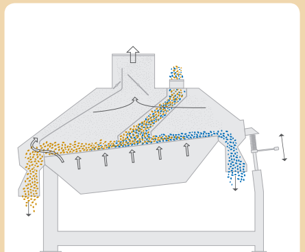
Schéma funkce
