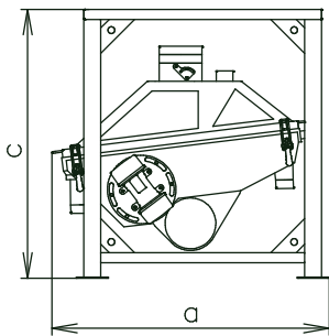
Rozměrové schéma
